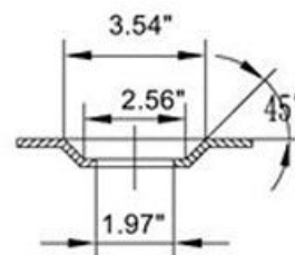
A-A 4:1
