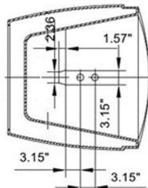
B2-B2
